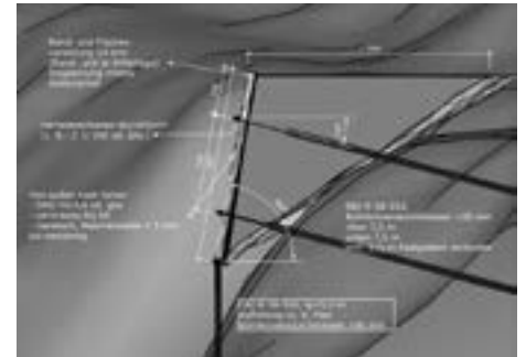
Systemskizze Ankerwand
